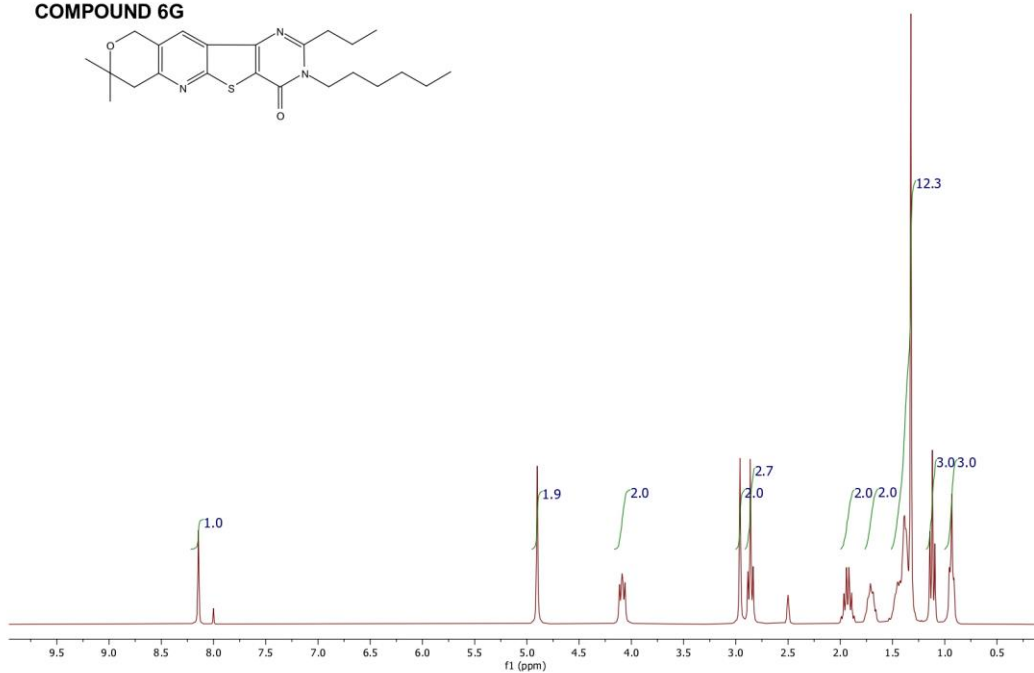
COMPOUND 6G
