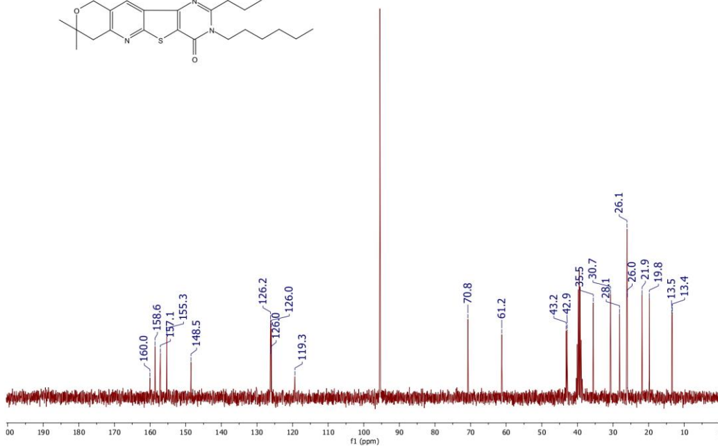
COMPOUND 6G
