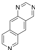
Pyrido[3,4- g ]quinazolines
