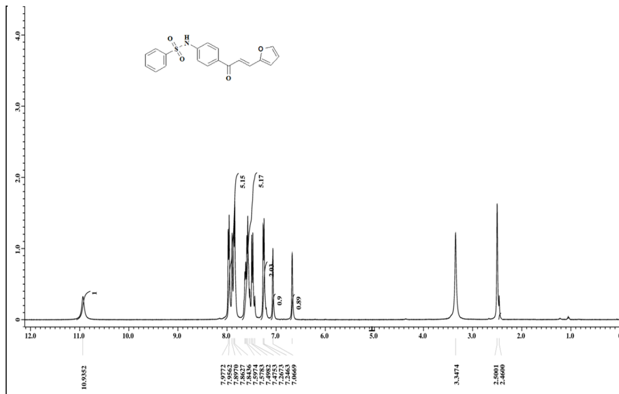
Fig. S11. 1 H spectrum of N -(4-(3-(furan-2-yl)acryloyl)phenyl)benzenesulfonamide (5f)
