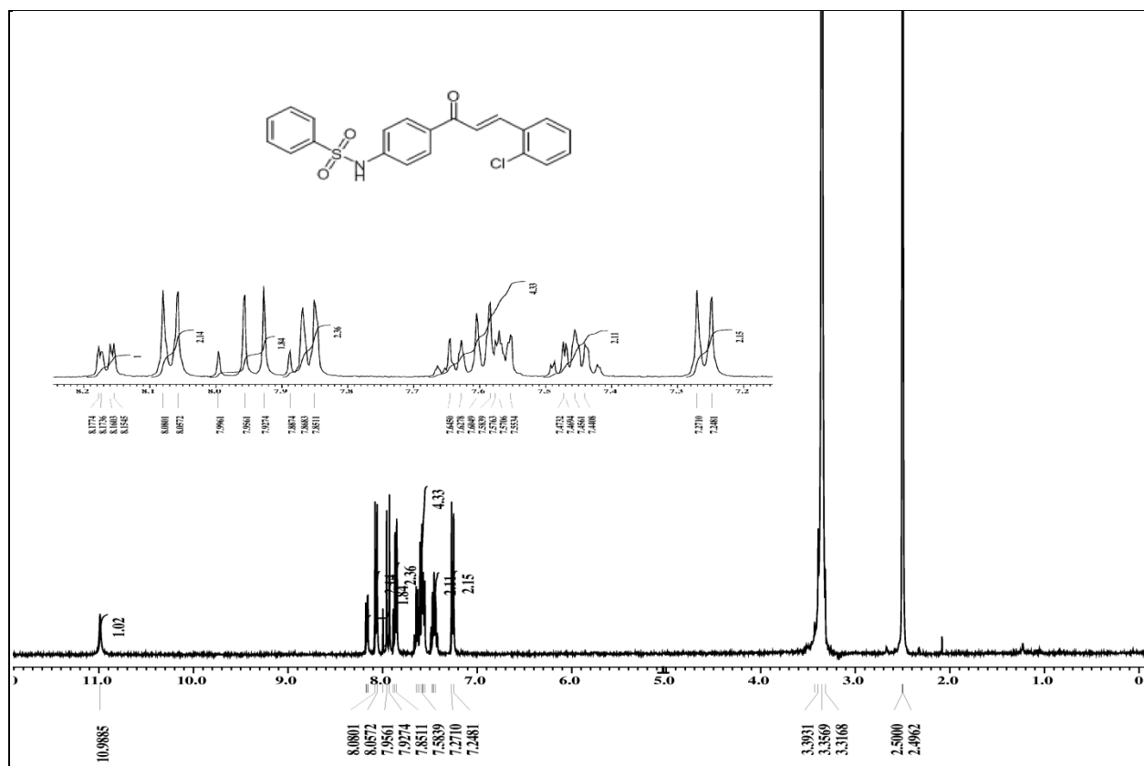
Fig. S15. ^1\text{H} spectrum of N -(4-(3-(2-chlorophenyl)acryloyl)phenyl)benzenesulfonamide (5h)
