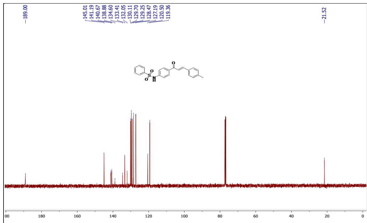
Fig. S20. ^{13}\text{C} spectrum of N -(4-(3-( p -tolyl)acryloyl)phenyl)benzenesulfonamide (5j)
