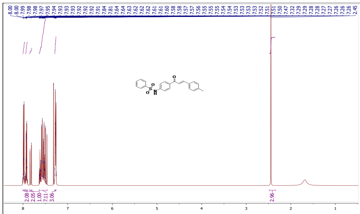
Fig. S19. ^1\text{H} spectrum of N -(4-(3-( p -tolyl)acryloyl)phenyl)benzenesulfonamide (5j)
