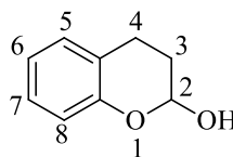
2-chromanol 1
