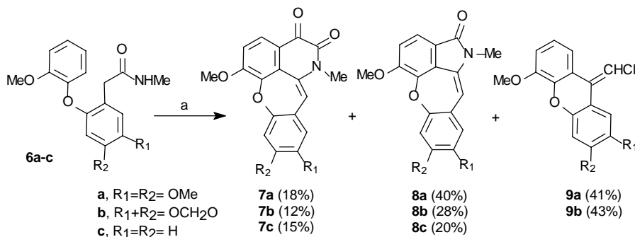
Scheme 3. (a) 1) (COCl) 2 /CH 2 Cl 2 ; 2) SnCl 4 /CH 2 Cl 2 .
