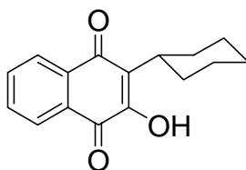
Parvaquone (1)
